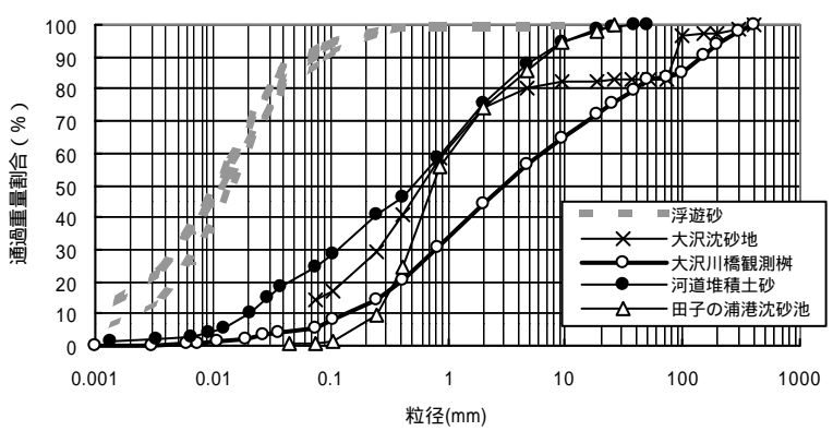
図 - 3 浮遊砂・掃流砂の粒度分布
